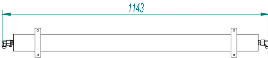
MEMBRANE CONTAINER SET
